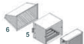
Caisson de mélange, et Plénum anti-pluie
